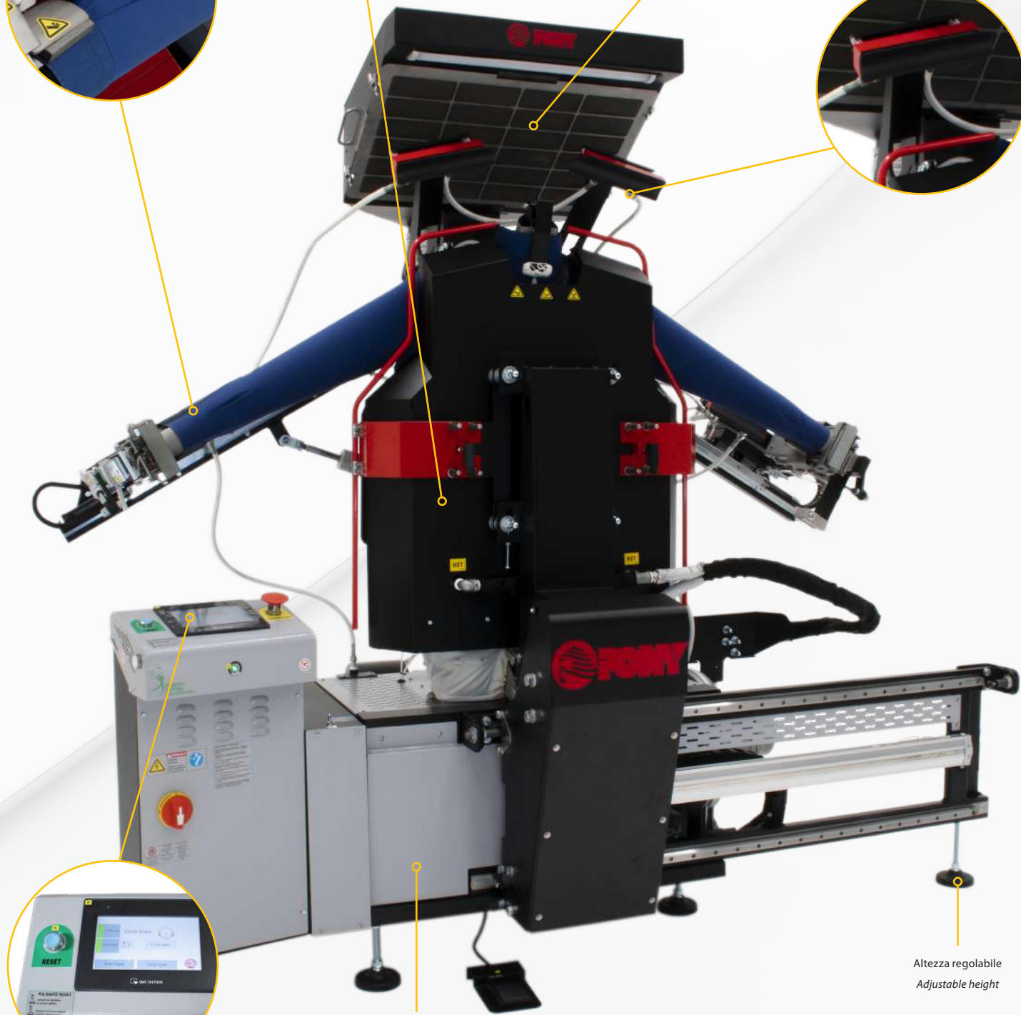
Struttura robusta e compatta Solid and compact framework
